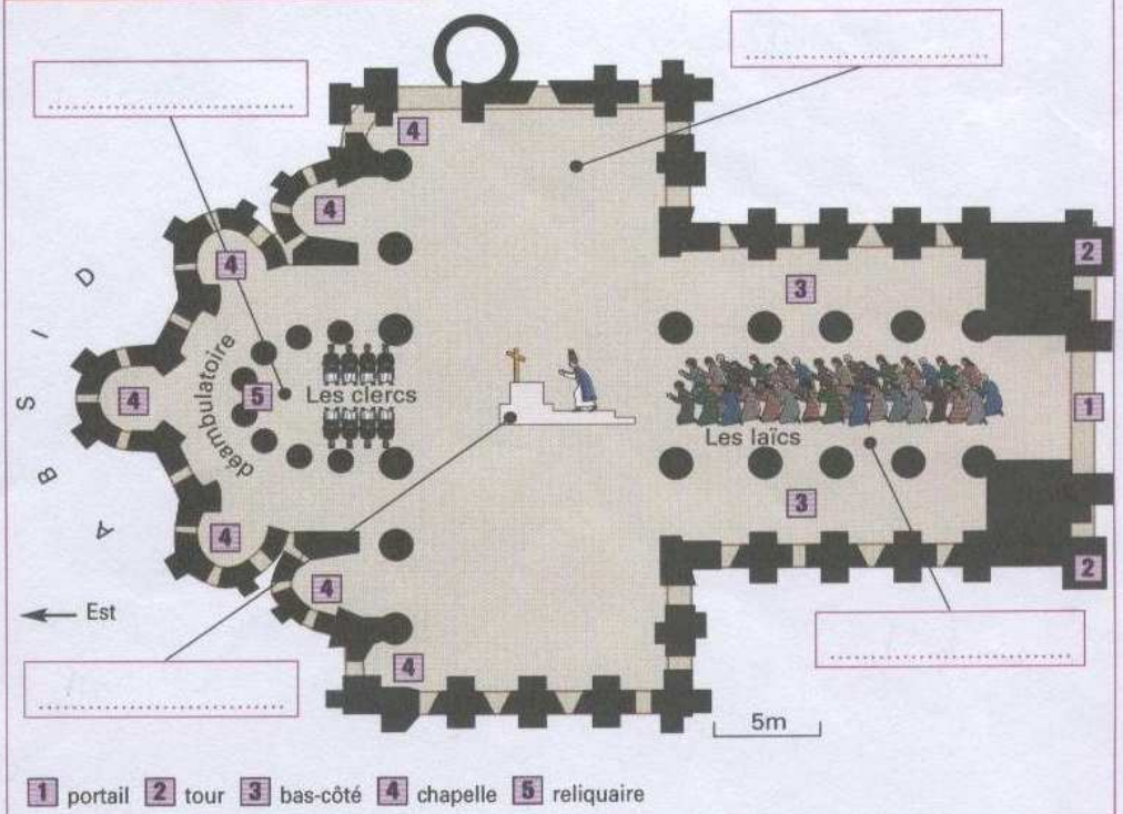
Plan de l'église Sainte-foy de Conques
